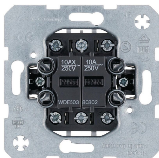
BERKER Serien Wechsel links Schalter/ rechts Taster, 10 A, Up
