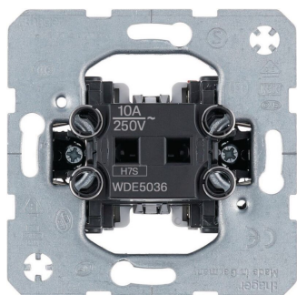
BERKER Wipptaster Einsatz mit Wechselkontakt, 10 A, Up
