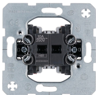
BERKER Doppelaster Einsatz, mit Öffner/ Schließer, getr. Meldekontakte, 10 A, Up
