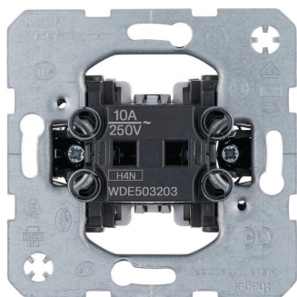
BERKER Serientaster 1 Öffner, 1 Schließer getrennte Eingangsklemmen, 10 A, Up
