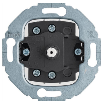
BERKER Serie 1930 Kreuzschalter Drehschalter, Kreuz, S 1930/Glas/R.classic
