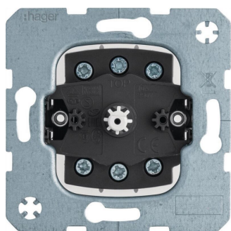
BERKER Jalousie-Drehschalter Tastrast-Funktion, 2polig
