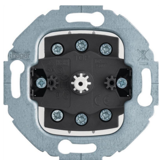
BERKER Serie 1930 Gruppentaster 2polig, 0-Stellung, getr. Eingangskl.
