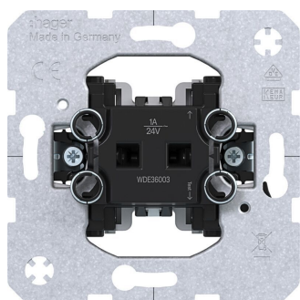
BERKER Wechselschalter 2 A, 24V, UP
