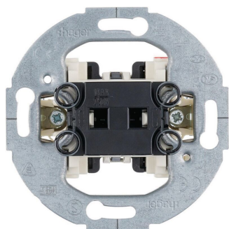
BERKER Wechselschalter Tragringschalter, Wipp-Einsatz, 10 AX, UP
