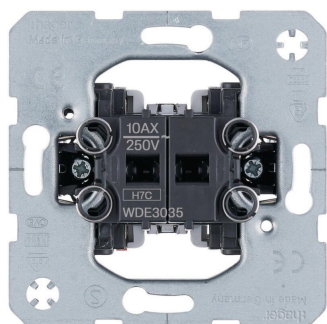
BERKER Serienschalter, Wipp-Einsatz 10 AX, Up
