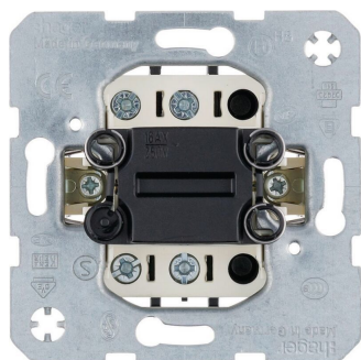
BERKER Ausschalter 2polig, Wipp-Einsatz, 16 AX, UP
