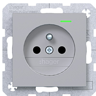
BERKER A.x/C.x SD, Schuko-sti. Kont. LED erh. Ber.schutz, Liftkl., titan m. lack.
