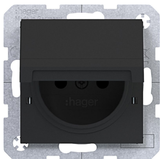
BERKER A.x/C.x SD Klapp arret Schuko-sti erh. Ber.schutz, Liftkl., n.schwarz m.
