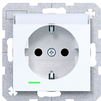
BERKER A.x/C.x SSD m. Kont.-LED, Besch. erh. Ber.schutz., Liftkl., lichtweiß. gl.
