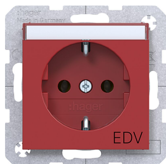
BERKER A.x/C.x SSD mit Aufdruck EDV, erh. Ber.schutz, rot glänzend
