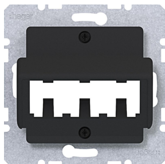
BERKER A.x/C.x Zentralplatte für 3 MINI-COM Module, nachtschwarz matt
