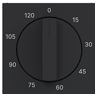
BERKER A.x/C.x Zstk. für 120 min. Zeitschaltuhr, nachtschwarz matt
