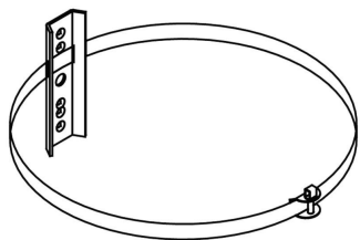
WHD Mastbefestigung MB 1/2 für TL5/TL6/T
