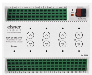
ELSNER KNX Aktor 4 Multifunktions-Ausg., 10 Eingänge
