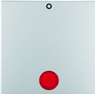
BERKER S.1 IP44 Wippe mit Befestigungss. mit Aufdruck 0 u. Linse alu matt
