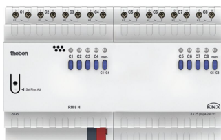
THEBEN KNX FIX Hochleistungsschaltaktor 8-fach, 25 A, 200 µF C-Last, RM8H, REG
