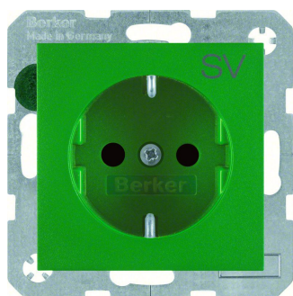
BERKER S.1/B.x SSD mit erhöhtem Berührungsschutz grün matt
