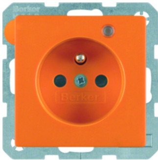
BERKER Q.x Steckdose mit Schutzkontakt und Kontroll-LED orange samt
