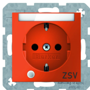
BERKER S.1/B.x SSD mit Kontroll-LED, BSF und Aufdruck "ZSV" orange matt
