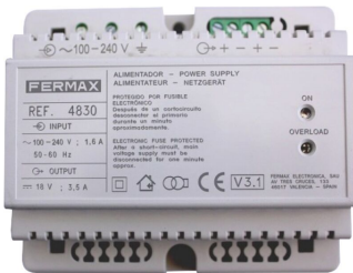
FERMAX Audio/Video Netzgerät, VDS 240Vac/18VDC-3,5A, TE6
