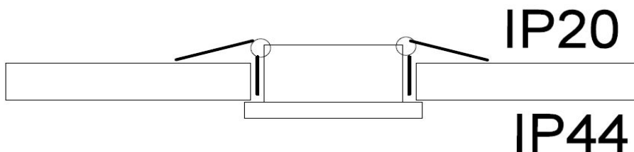
Abbildung 3 Einbau in geschlossene Decken
