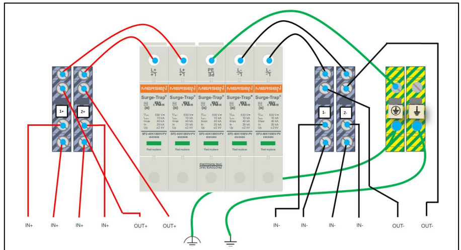
Anschlusszeichnung
