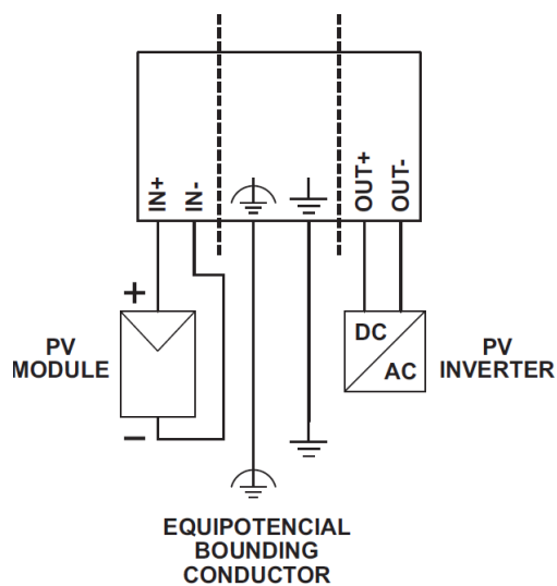
Anschlusszeichnung
