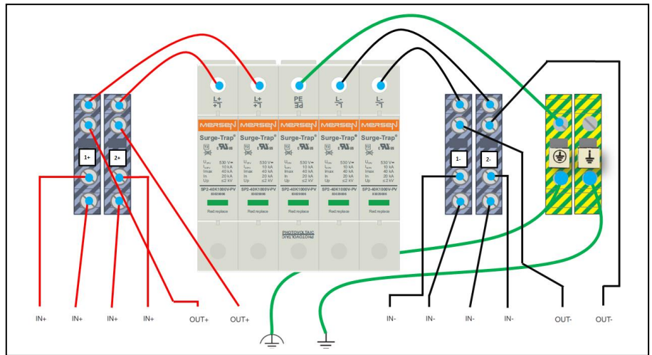
Anschlusszeichnung
