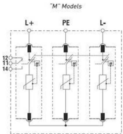
Überspannungsschutz - Prinzipschaltbild
