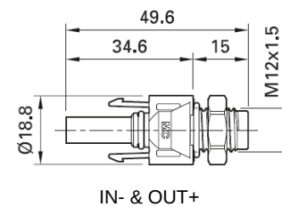
MC4 Stecker
