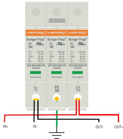
Anschlusszeichnung
