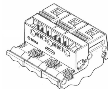
2 Mikroschalter CMS22W3
