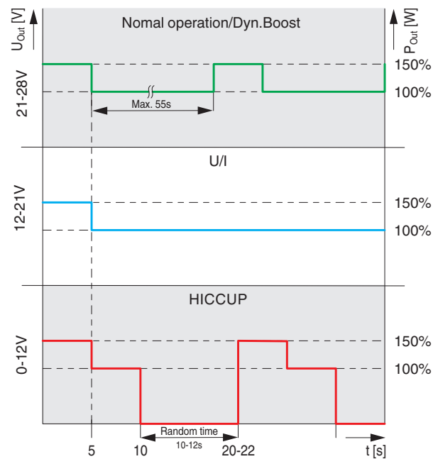
Bild 40 Ausgangskennlinien abhängig vom DC-Lastverhalten
