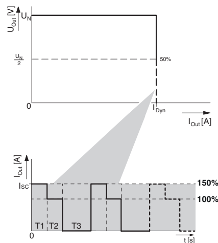
Bild 42 Prinzipdarstellung HICCUP-Ausgangskennlinie
