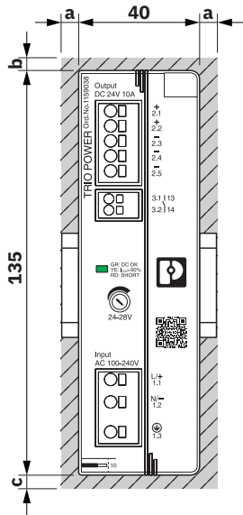
Bild 11 Geräteabmessungen und minimale Sperrflächen (Maße in mm)
