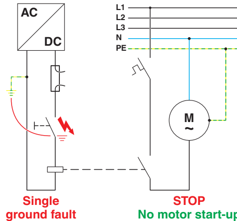
Bild 30 Prinzipdarstellung mit sekundärseitiger Erdung
