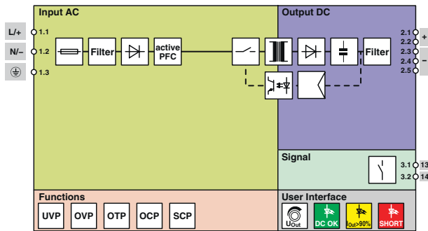
Bild 6 Blockschaltbild
