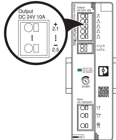
Bild 26 Lage der DC-Ausgangsklemmen
