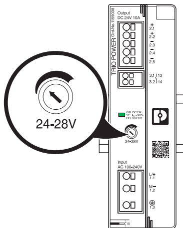
Bild 36 Lage des Potenziometers
