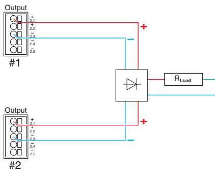
Bild 45 Prinzipdarstellung, 1+1-Redundanz mit Redundanzmodul (aktiv oder passiv)
