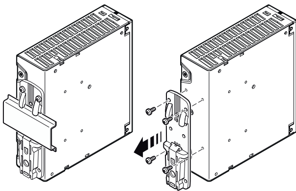
Bild 14 Universal-Tragschienenadapter demontieren
