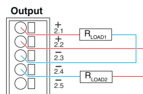
Bild 27 Prinzipbeschaltung der DC-Ausgangsklemmen
