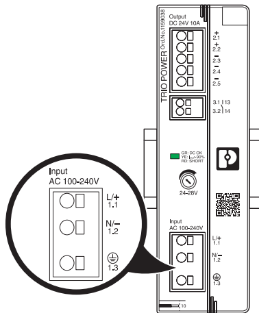
Bild 22 Lage der AC-Eingangsklemmen
