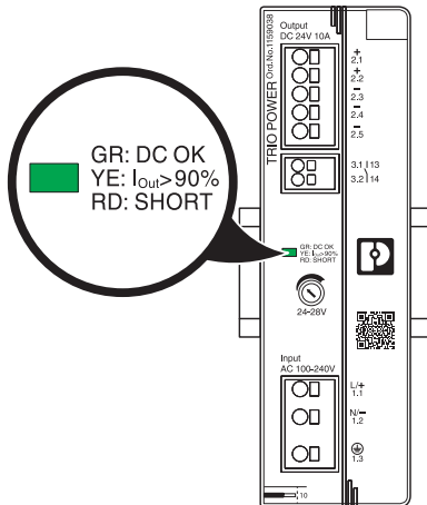
Bild 39 Signalzustände der DC OK-LED (Multicolor-LED)
