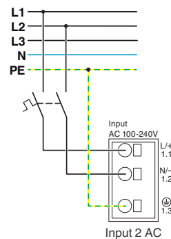
Bild 24 Prinzipdarstellung, 2-polige Absicherung
