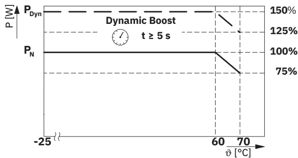
Bild 46 Ausgangsleistung in Abhängigkeit zur Umgebungstemperatur
