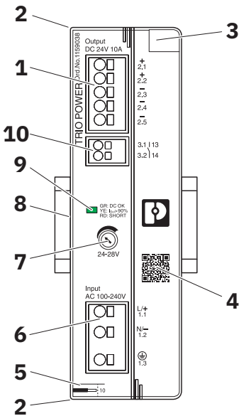
Bild 5 Lage der Anschlussklemmen und Funktionselemente
