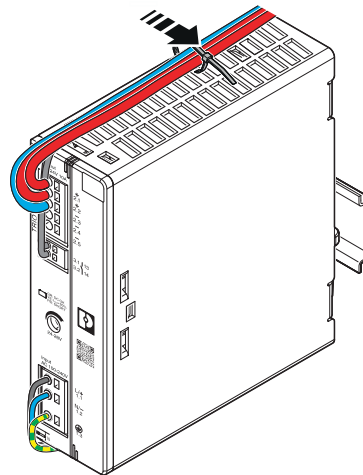
Bild 34 Anschlussleitungen bündeln und fixieren
