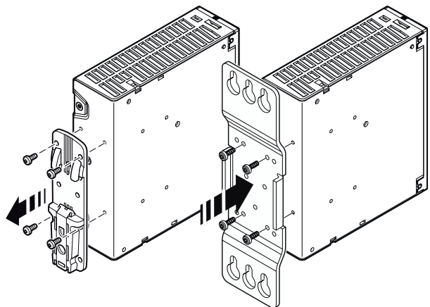
Bild 17 UWA 182/52 auf linker Gehäuseseite montiert
