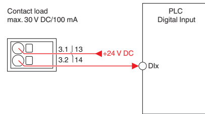
Bild 32 Prinzipbeschaltung des potenzialfreien Schaltkontakts
