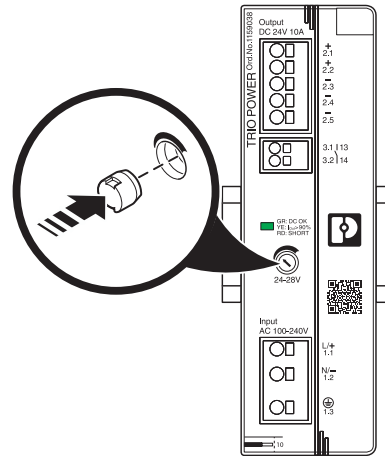
Bild 37 Verschlussstopfen stecken
