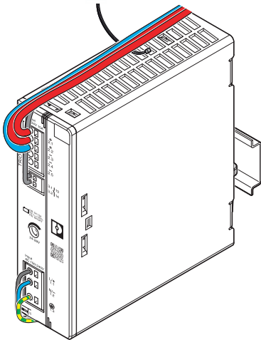
Bild 33 Anschlussleitungen verlegen und ausrichten
