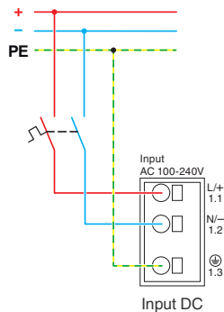
Bild 25 Prinzipdarstellung, 2-polige Absicherung
