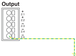
Bild 28 Prinzipbeschaltung der zusätzlichen Minusklemme
