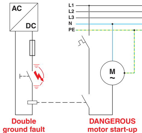
Bild 29 Prinzipdarstellung doppelter Erdschluss
