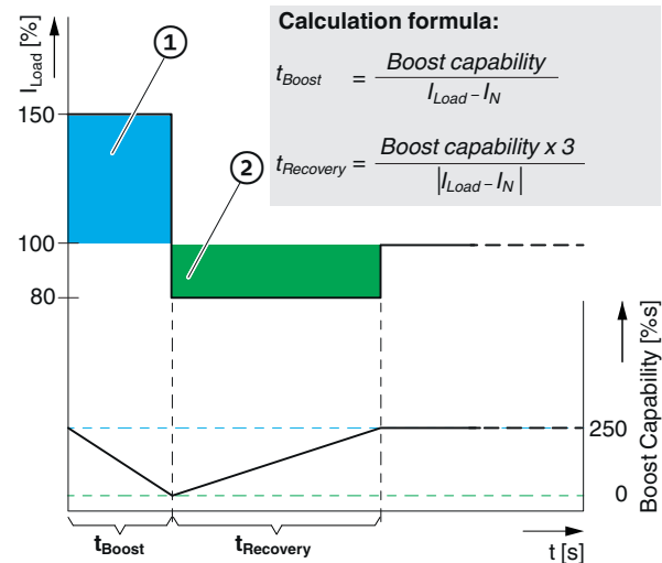
Bild 41 Allgemeine Darstellung und Berechnungsgrundlage, dynamischer Boost
