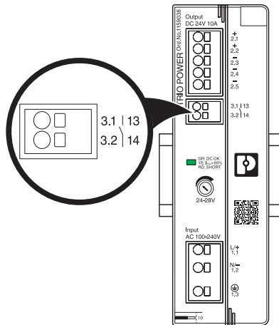
Bild 31 Lage des potenzialfreien Schaltkontakts
