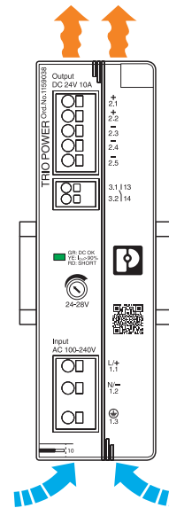
Bild 9 Prinzipdarstellung der Konvektionskühlung
