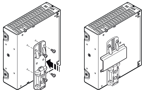
Bild 15 Universal-Tragschienenadapter montieren
