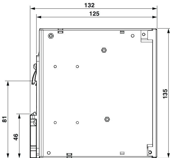
Bild 8 Abmessungen Seitenansicht (Maße in mm)
