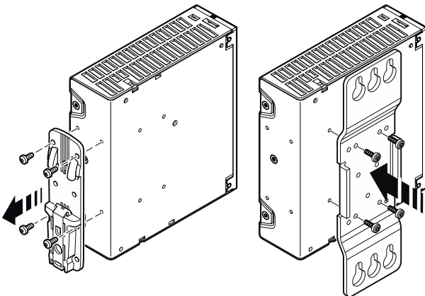
Bild 16 UTA 107/30 durch UWA 182/52 ersetzen
