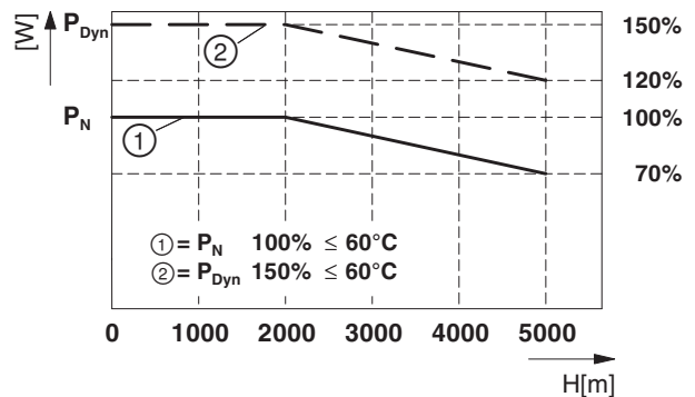
Bild 47 Ausgangsleistung in Abhängigkeit zur Aufstellhöhe
