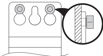
Bild 19 Prinzipdarstellung, Schraubbefestigung auf der Montagefläche
