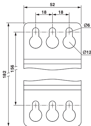
Bild 19 Prinzipdarstellung, Schraubbefestigung auf der Montagefläche
