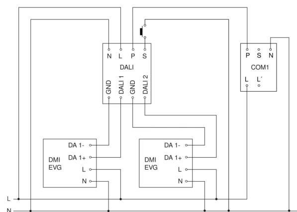
Schaltplan Master-Master Vernetzung
