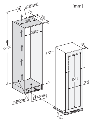
KWT6722iS, KWT6722iS-1, Skizze
