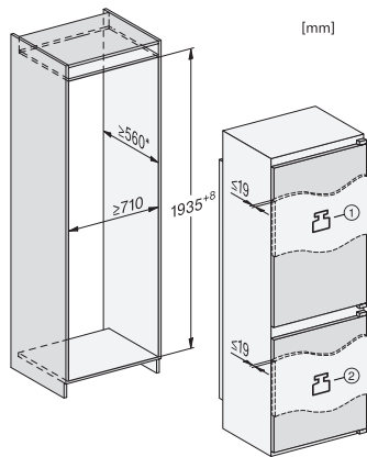
KFN7934D, Einbau
