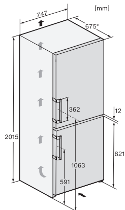
KFN4796AD, KFN4796CD, KFN4796ED, Aufstellskizze
