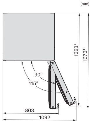
KFN4776ED, KFN4776ED C, KFN4796AD, KFN4796CD, Draufsicht
