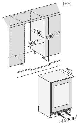
KWTUS7196E, Built-under, Einbauskeizze, Nischenmaß (Skizze)
