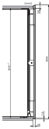
KWT6422iG, KWT6422iG-1, Seitenansicht (Skizze)
