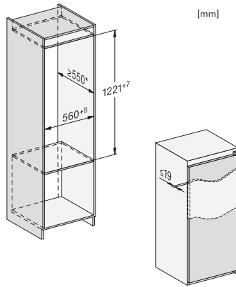
K7318D, K7328D, K7316E, K7326E, K7317D, K7327D, K7315E, K7325E, Einbau (*Fußnote) (Skizze)
