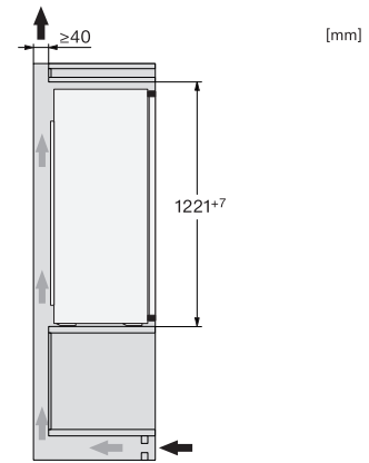
K7318D, K7328D, K7316E, K7326E, K7317D, K7327D, K7315E, K7325E, Seitenansicht (Skizze)
