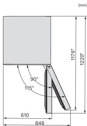
KFN4898CD, KFN4795DD bb Blackboard, Draufsicht (*Fußnote) (Skizze)
