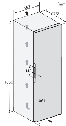
FN4872D, FN4874C, KS4887DD, Aufstellskizze (*Fußnote) (Skizze)
