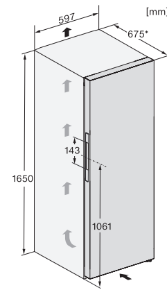
FN4842D, FN4844C, Aufstellskizze (*Fußnote) (Skizze)
