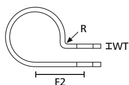
Aluminiumschelle (Seitenansicht)
