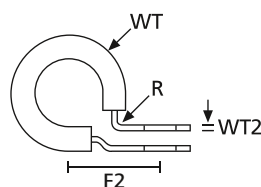
Aluminiumschelle mit Chloroprenschutzprofil (Seitenansicht)
