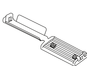
Befestigung wahlweise mit Acrylat-Klebeband oder M3-Schrauben
