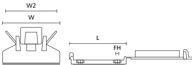
Kabelhalter für Flachbandkabel (Frontansicht)
