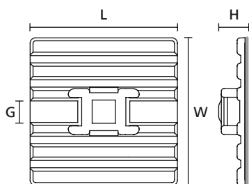
Flexibler Klebesockel FMB4APT-A (Draufsicht)
