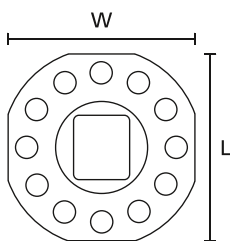
PMB5 Sockel (Draufsicht)
