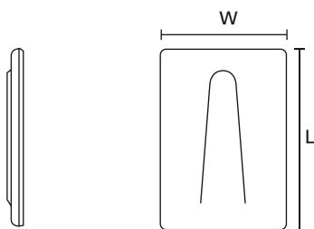
Befestigungssockel SAC-Serie
