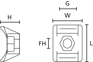
NY3256 (Seitenansicht)
