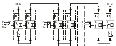
Prinzipschaltbild
