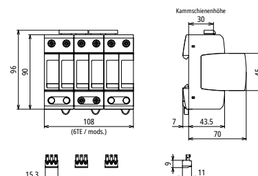
Maßbild
