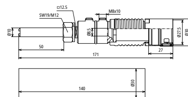
Maßbild
